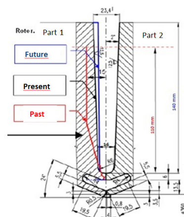
Figure 1. „ultra“ Narrow Gap
